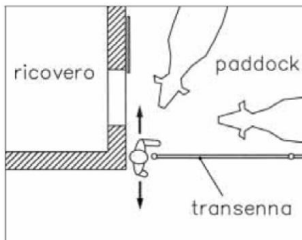
Figura 62: Progettazione di vie di fuga per gli operatori.
