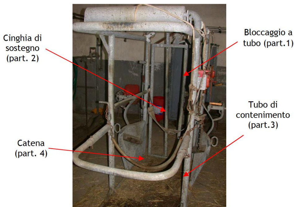
Figura 77: Travaglio per bovini.
